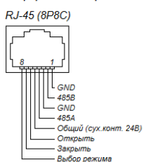
Интерфейсный разъём
