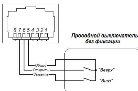
Управление по "сухим" контактам
