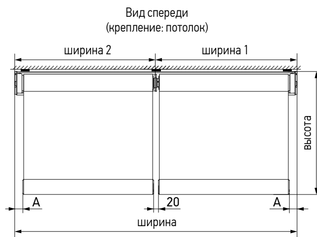
Габаритные размеры. DOUBLE AMG
