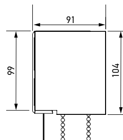
Вид сбоку
