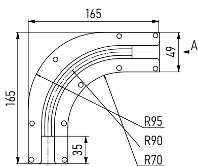
Соединитель карнизов 90 гр
