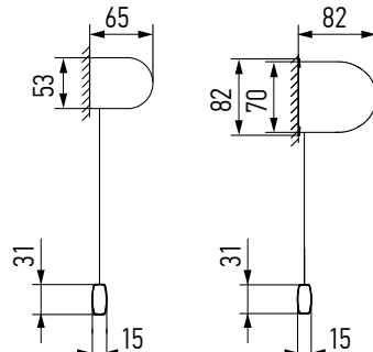
Вид сбоку (крепление: стена)
