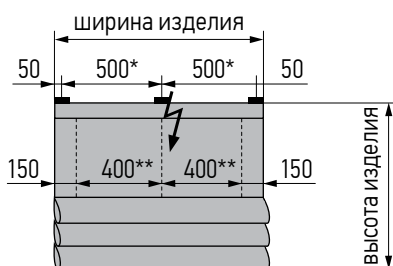
Вид спереди
