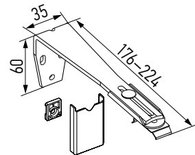
Кронштейн стеновой регулируемый 156-204 мм
