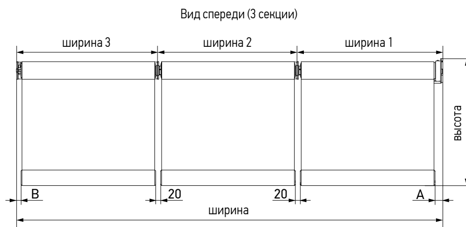
Габаритные размеры. MONO AMG
