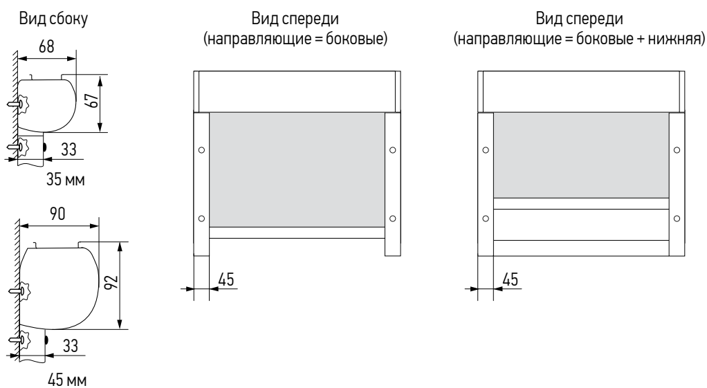
Габаритные размеры. Кассета AMG. Опция направляющие. На проем
