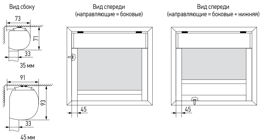
Габаритные размеры. Кассета AMG. Опция направляющие. В проем
