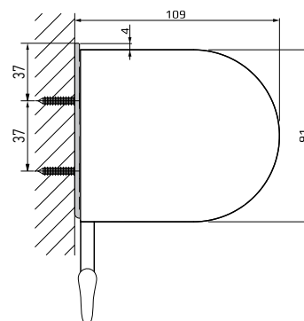
Вид сбоку
