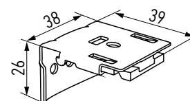
Кронштейн для римской шторы пружинный 530104-0225
