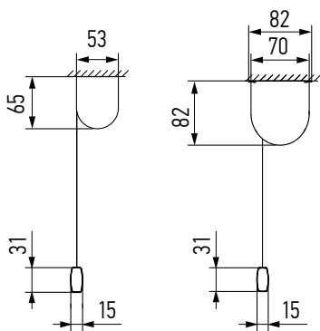
Вид сбоку (крепление: потолок)
